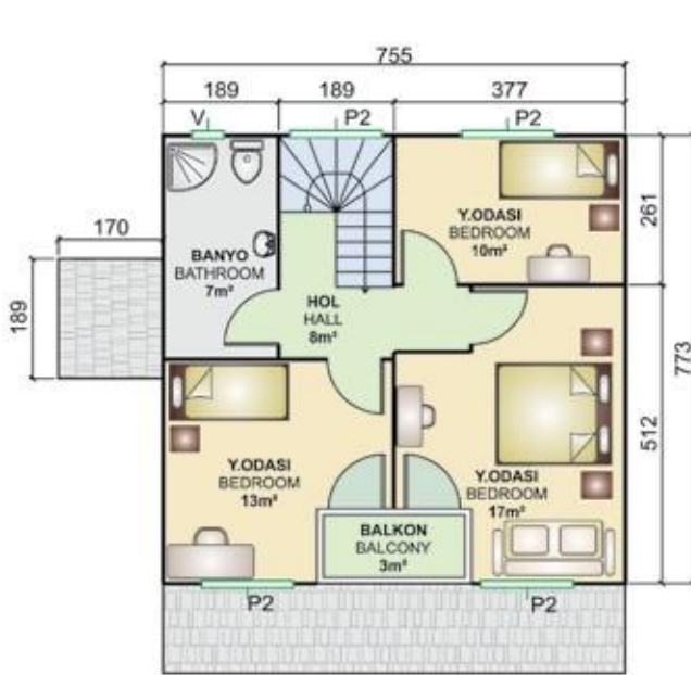
56 m 2 + 3 m 2 = 59 m 2 1.Kat Planı / First Floor Plan
