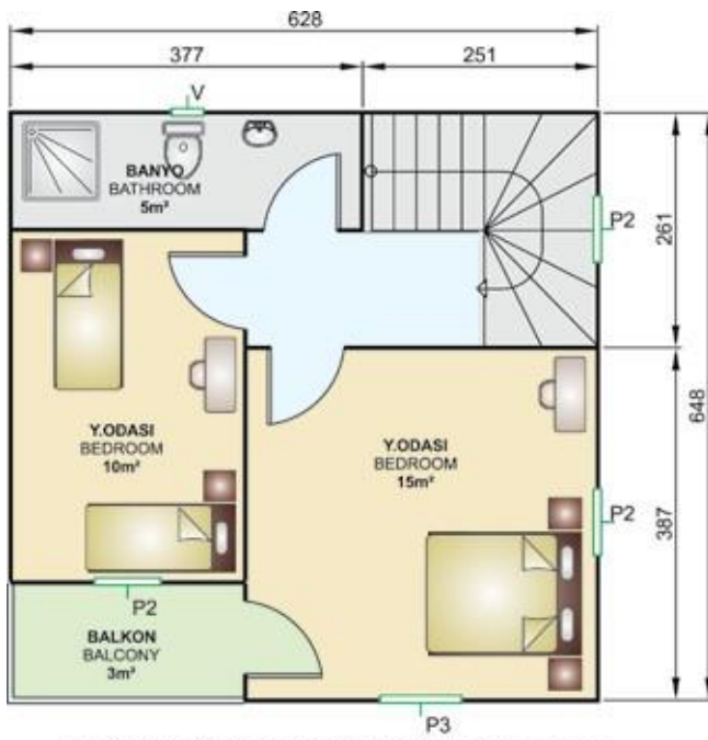
37 m 2 + 3 m 2 = 40 m 2 1.Kat Planı / First Floor Plan
